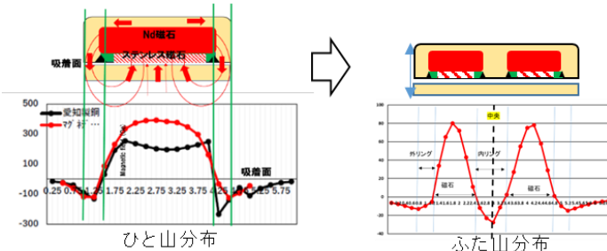
説明図 リング磁気回路構造で薄型化を実現
