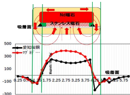
説明図 磁気回路構造
