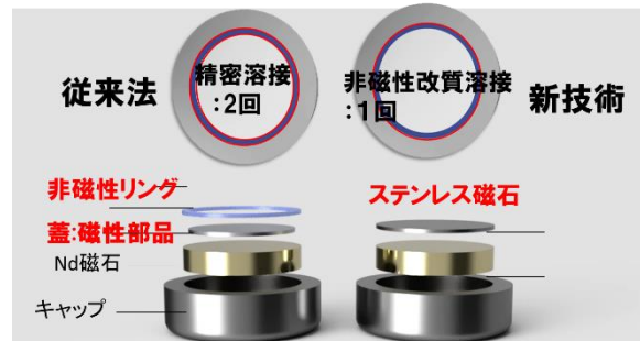
説明図 非磁性改質・溶接技術
